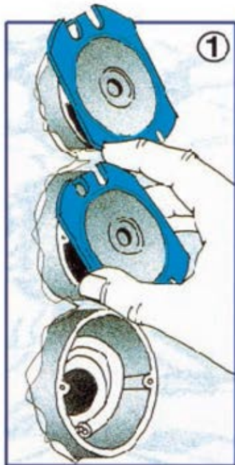
1 Asennetut sähkörasiat, jotka voivat olla kiinnitettyinä tai irrallaan, myös johdotettuina. Paina magneettipesä rasiaan ja asenna levy.
