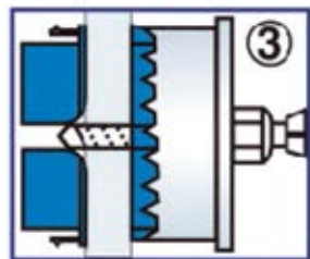
3 Pora reikä sahatyyppi H 97 kattoon ja H 75 seinään. Asenna keskiöpora 5 mm yli levyn paksuuden , siten saat täydellisen lopputuloksen.
